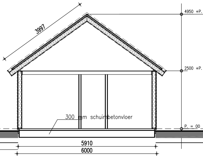
Doorsnede
