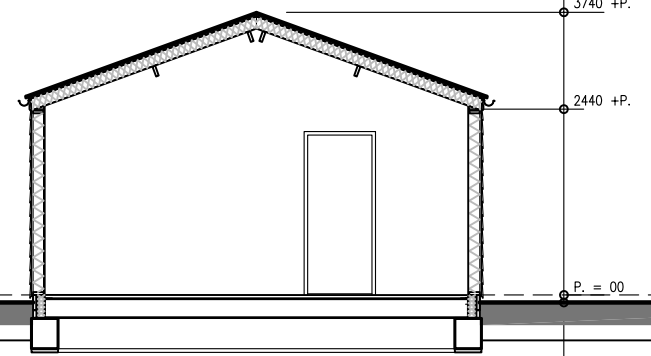
Doorsnede
