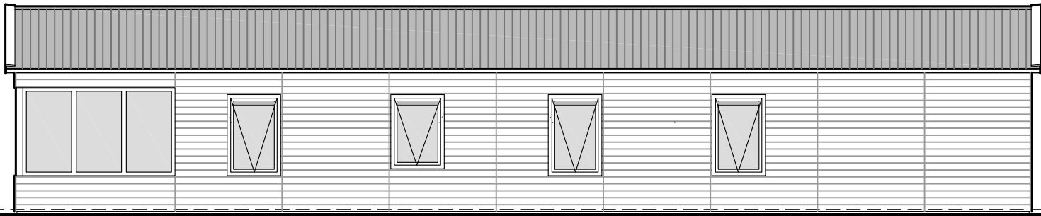
Achtergevel
