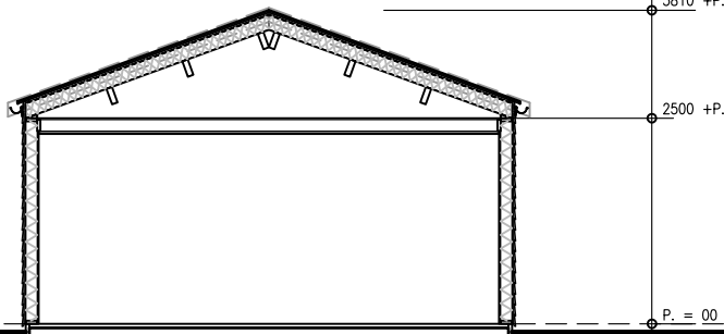
Doorsnede
