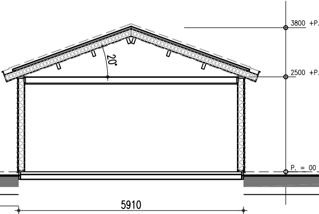
Doorsnede
