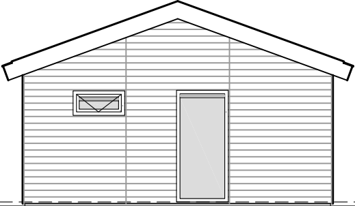
Rechter zijgevel
