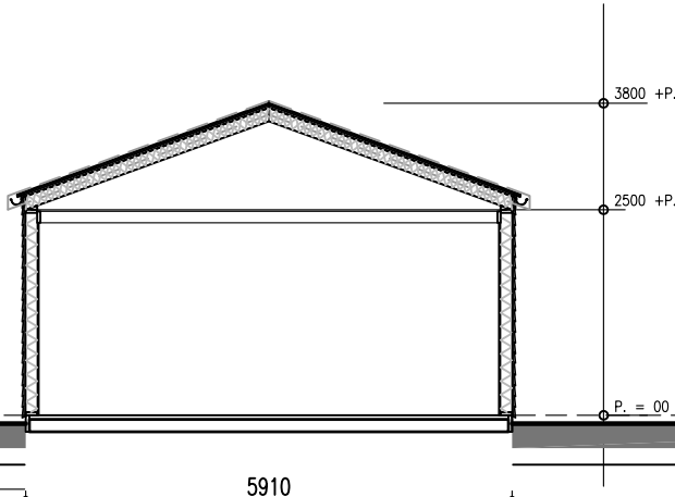
Doorsnede
