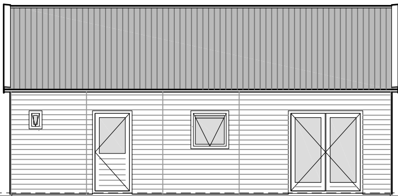
Voorgevel
