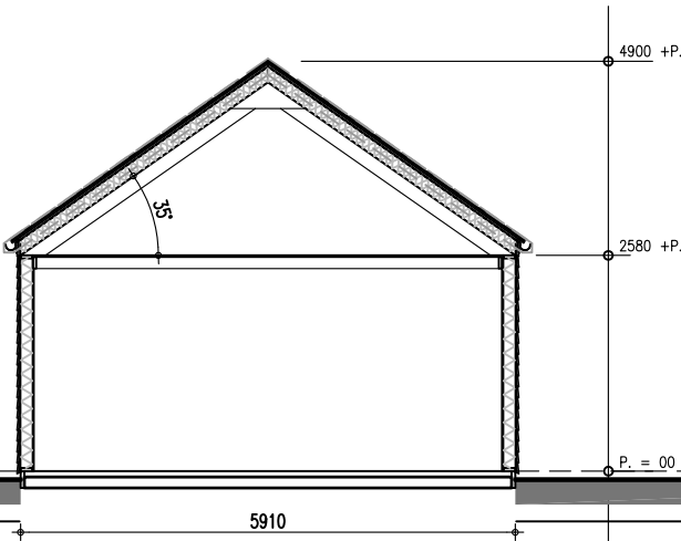
Doorsnede
