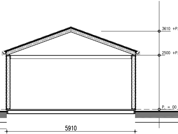
Doorsnede
