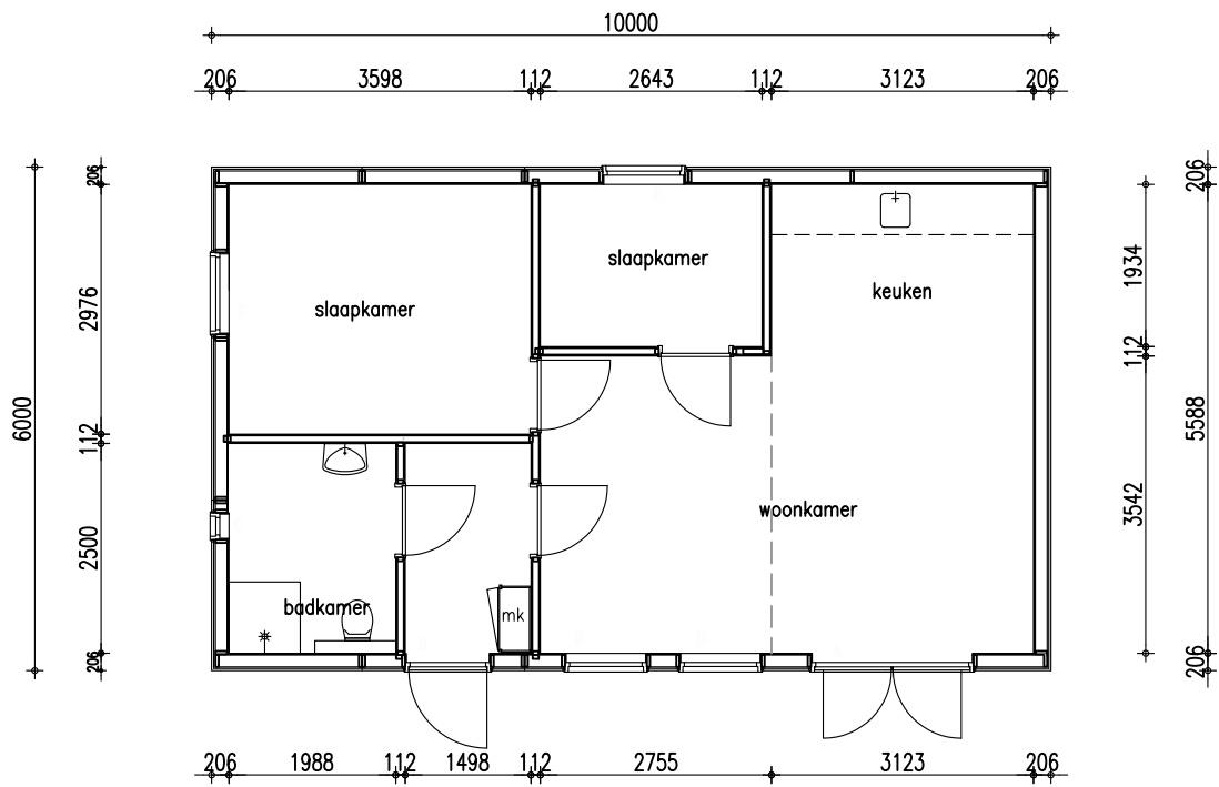
Beganegrond
