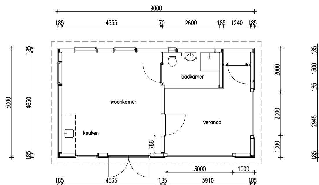
Beganegrond
