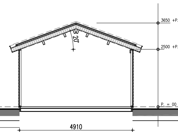
Doorsnede
