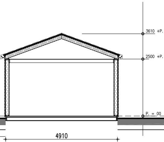
Doorsnede
