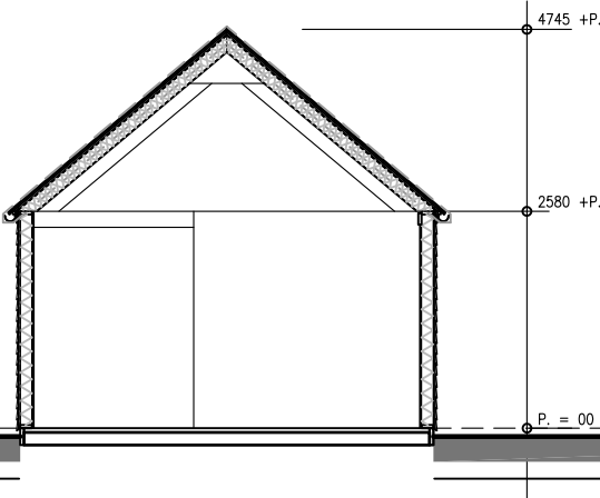
Doorsnede
