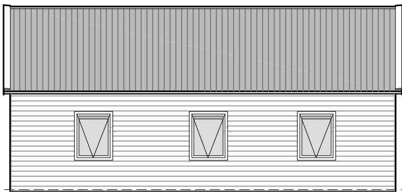
Achtergevel
