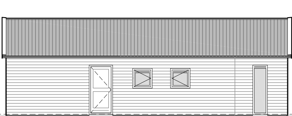
Voorgevel
