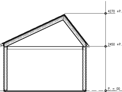
Doorsnede
