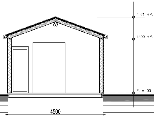
Doorsnede woonkamer
