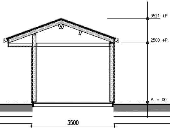
Doorsnede slaapkamer
