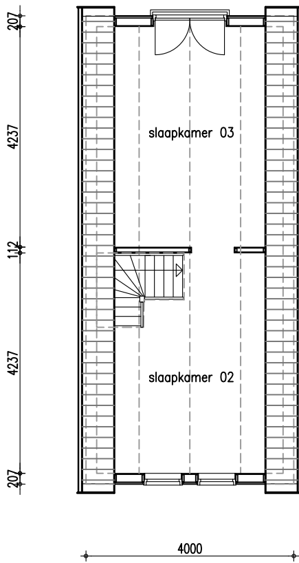
1e verdieping
