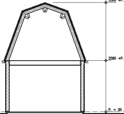
Doorsnede
