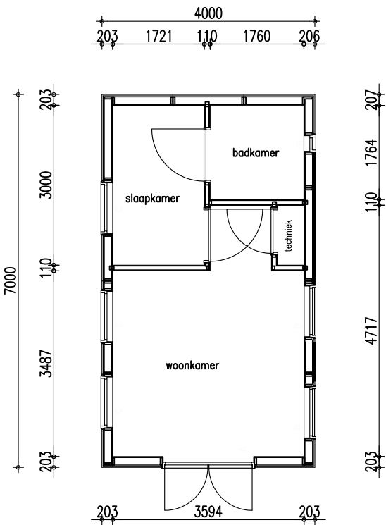
Beganegrond
