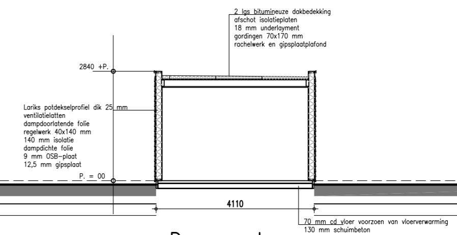
Doorsnede
