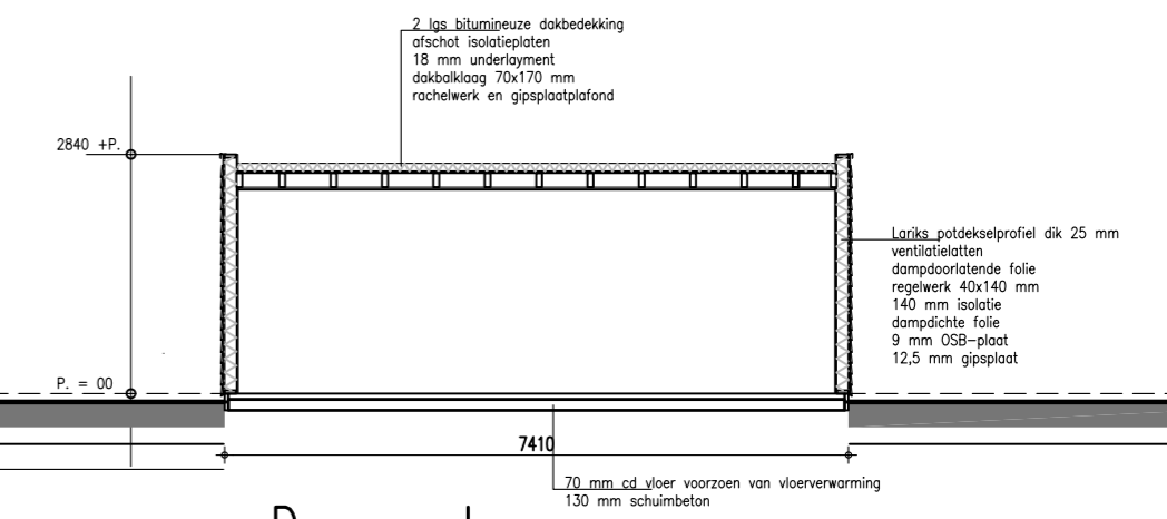
Doorsnede
